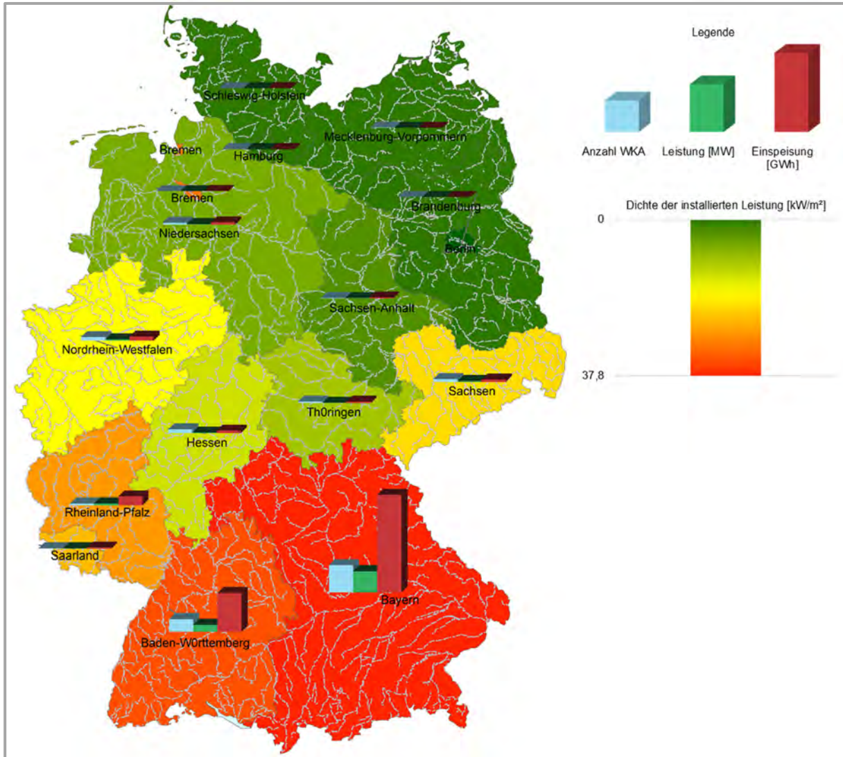
Abbildung 13: Übersicht der Wasserkraftanlagen (Anzahl, Leistung, Einspeisung) in Deutschland nach Bundesländern (Bundesnetzagentur, 2019; Länderarbeitskreis (LAK) Energiebilanzen, 2019 49 ; Arbeitsgruppe Erneuerbare Energien-Statistik beim Umweltbundesamt, 2018 50 )
