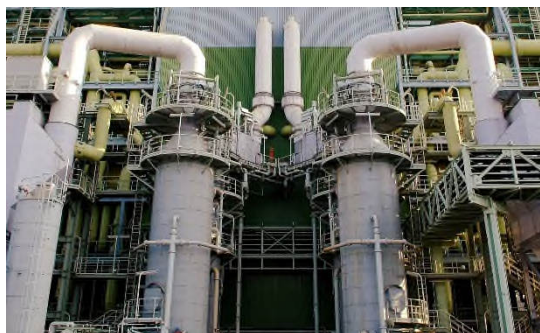
Klärschlammverbrennungsanlage im Industriepark Höchst
