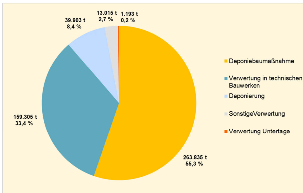
Abbildung 34: Entsorgungswege der Schlacken aus hessischen MCHP und EBS-Kraftwerken 2016 (Quelle: HMKLV, 2016)
